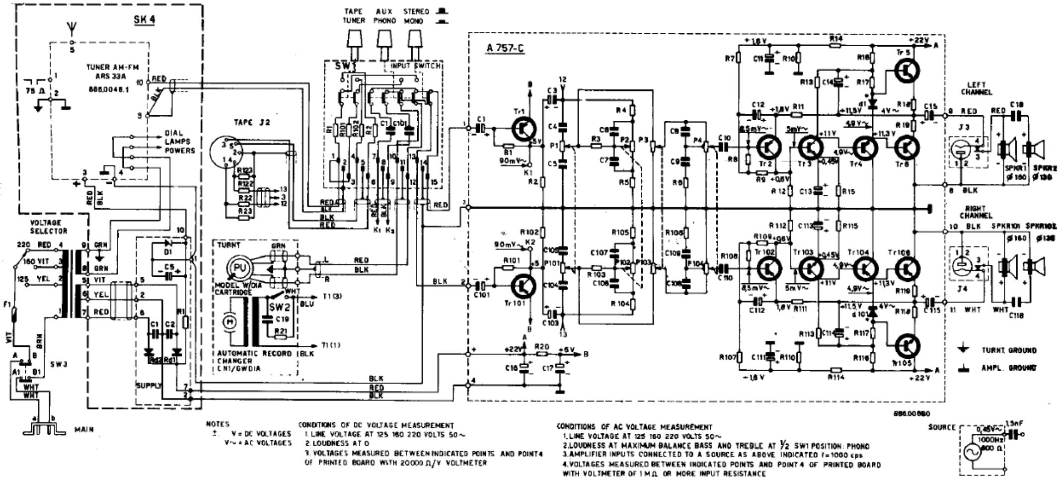
Schema elettrico LF 760/R
